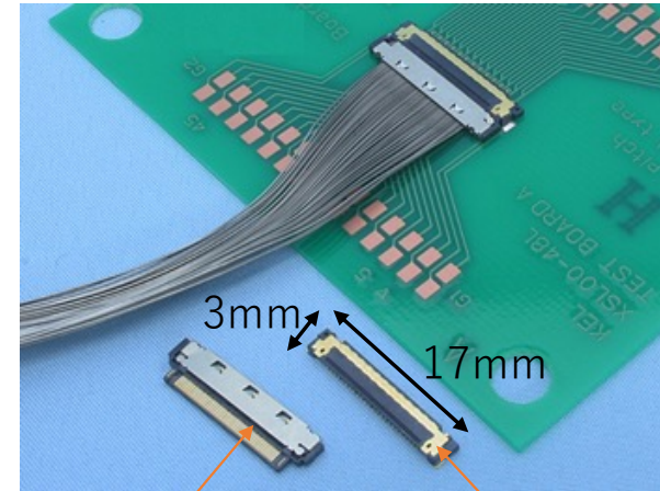
Cable end
