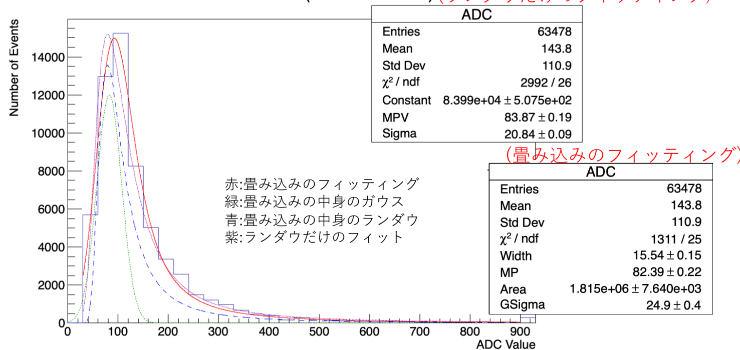
ADC Distribution (80 <math>< \theta </math> <math>< 90</math>) (ランダウだけのフィッティング)
