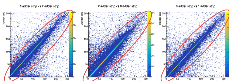
図 5.15 基準ラダーの相関分布
