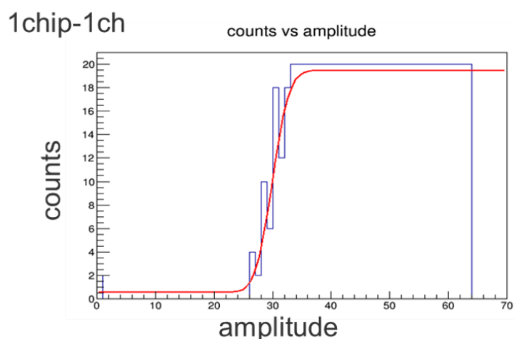
図 A.1 チップ1チャンネル1の入力波高ごとのヒット数分布
