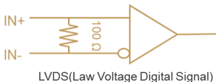
図 4.18 LVDS の回路図
