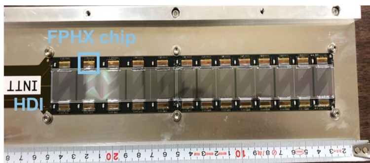
図 2.4 INTT ハーフラダー
