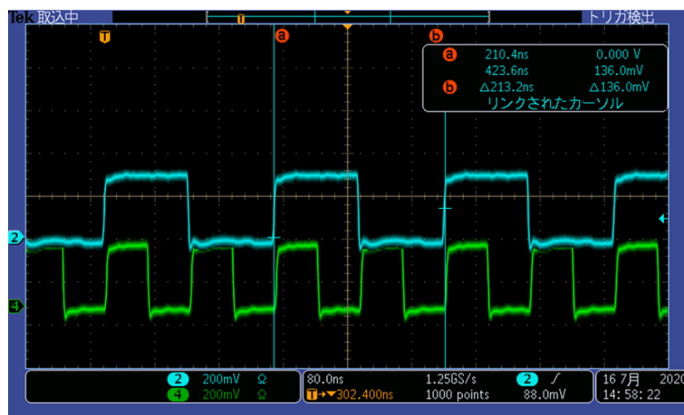
図 A.6 BCO と START の出力波形
