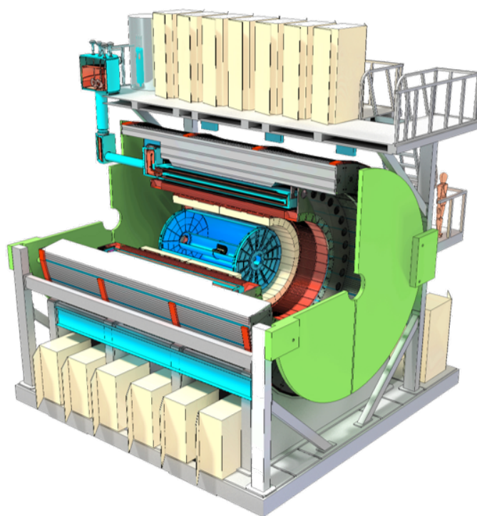
図 1.4 sPHENIX 測定器
