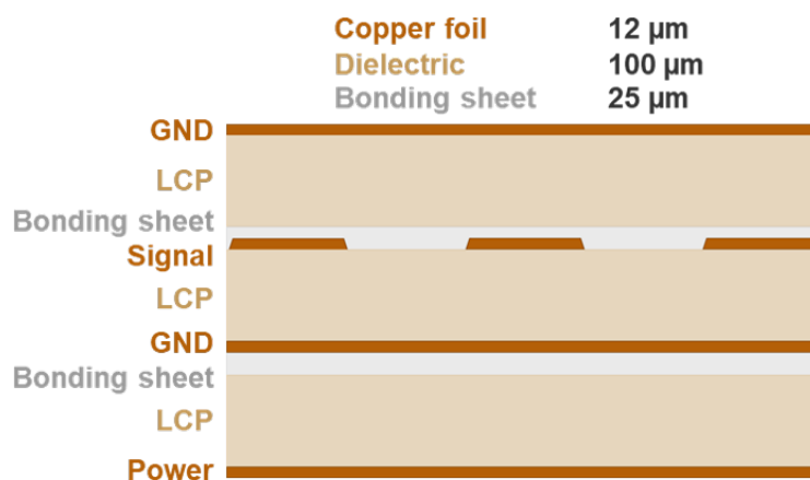
図 2.11 Bus-Extender ケーブルの層構造
