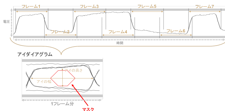
図 4.23 アイダイアグラムの作成
