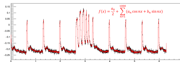
図 4.36 出力波形のフーリエ変換
