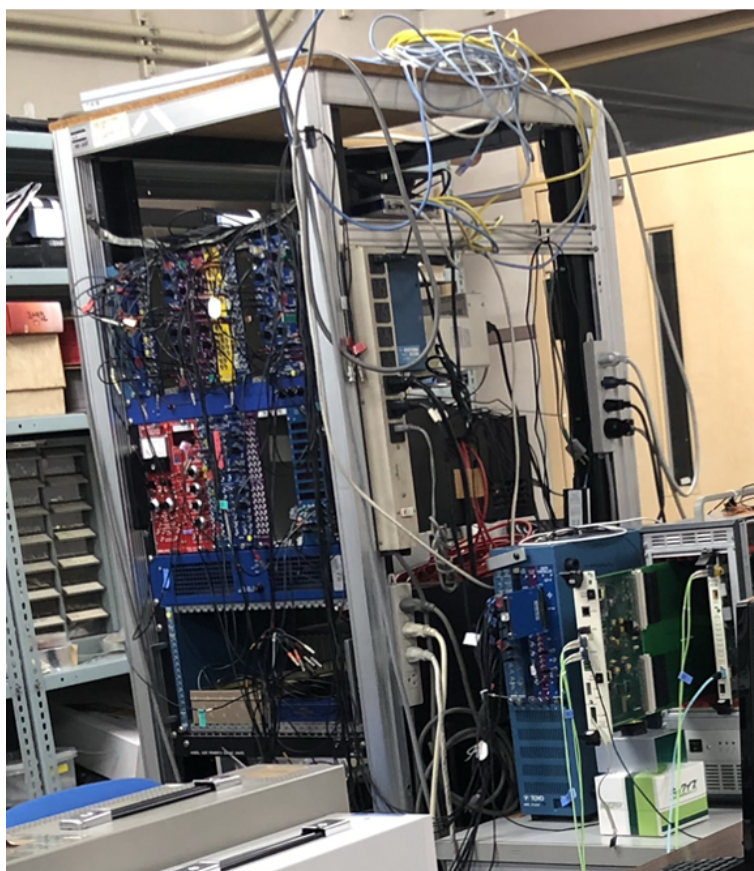
図 5.7 NIM と CAMAC
