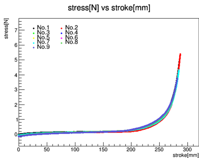
図 4.5 試験片を押した力と距離
