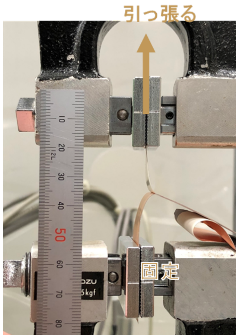
図 4.8 剥離試験
