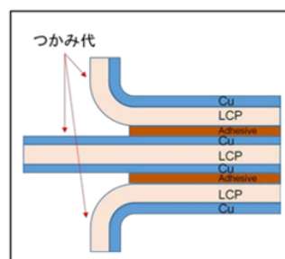
図 4.9 引き剥がす箇所
