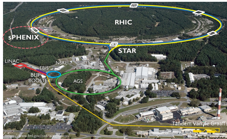
図 1.3 RHIC 加速器
