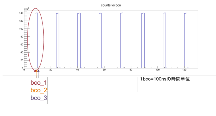
図 A.2 3回連続で来るヒット
