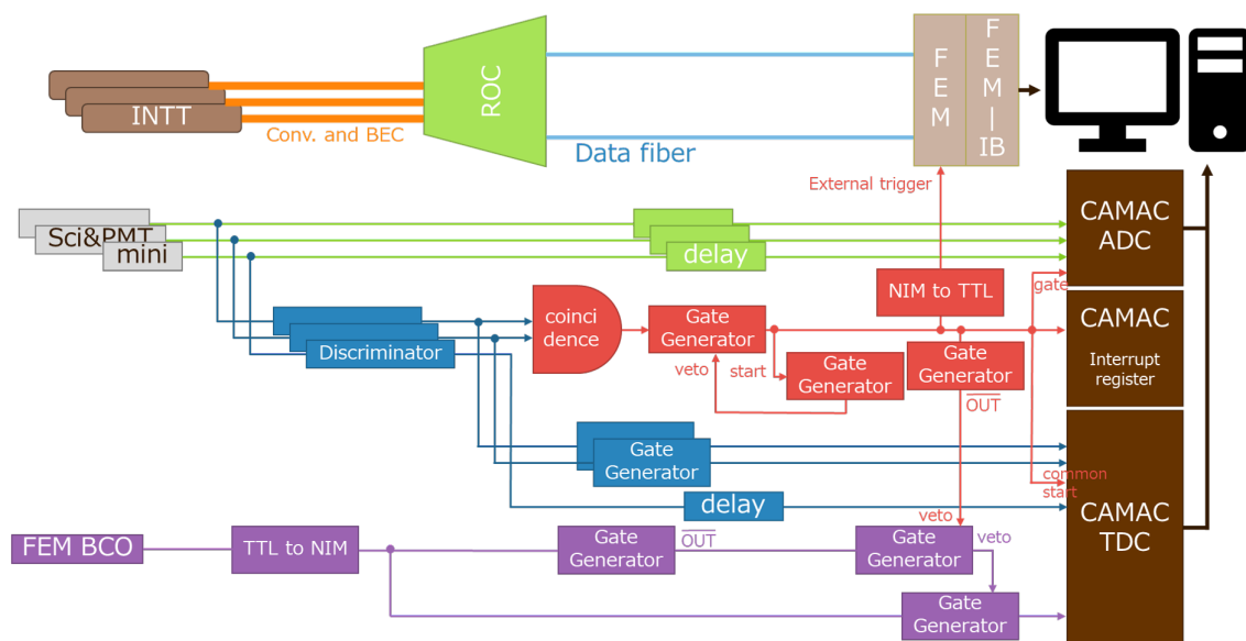
図 5.6 ビームテストの回路図
