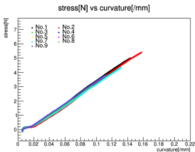
図 4.6 試験片を曲げる力に対する曲率
