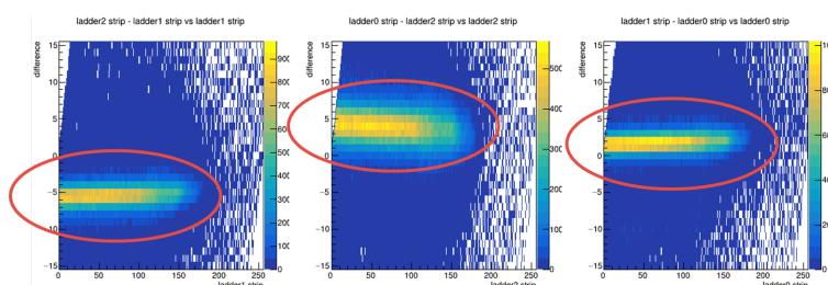
図 5.14 基準ラダーの差に対するクラスターヒット位置
