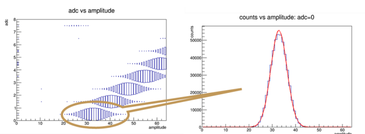
図 3.7 ADC と入力パルスの相関関係を示す分布
