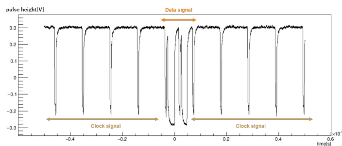
図 4.22 出力波形
