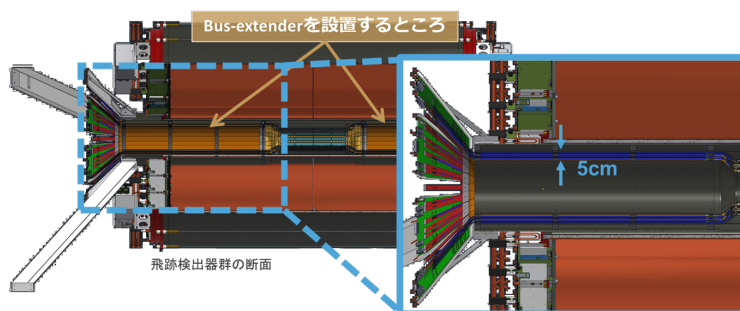
図 2.9 検出器群中の Bus-Extender の設置位置
