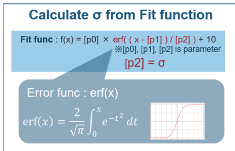
図 3.4 ノイズ評価を行うための Fit 関数
