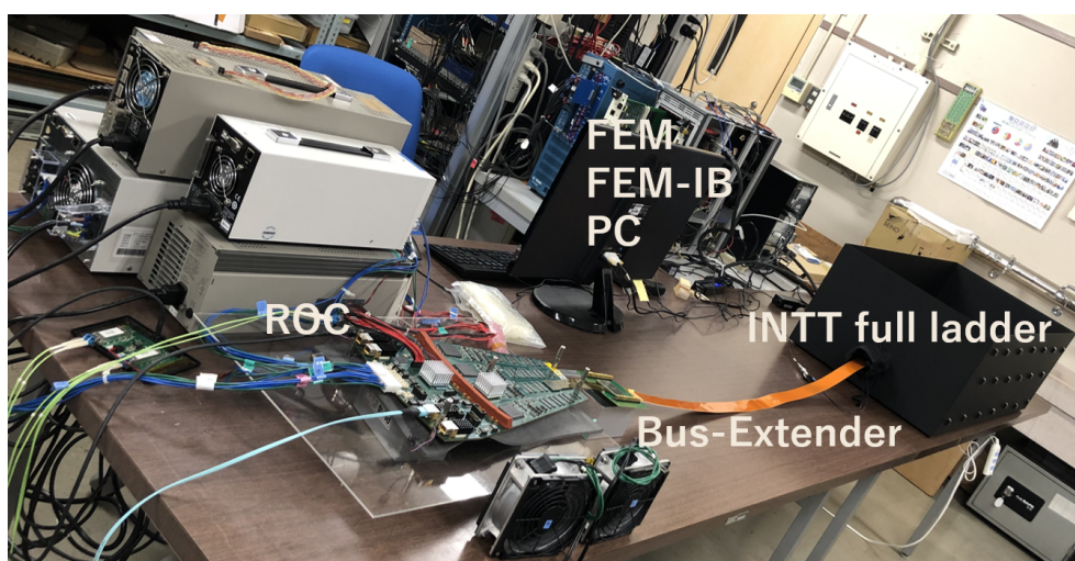
図 3.1 奈良女子大学のテストベンチ
