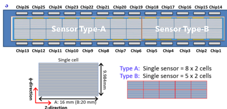
図 2.7 シリコンセンサー
