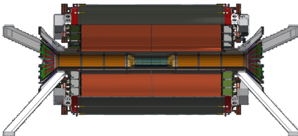
図 2.1 検出器群の断面
