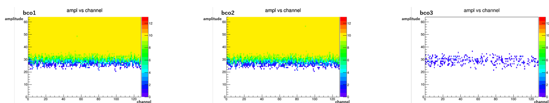
図 A.3 チップ1つ分のチャンネルごとの入力信号に対するヒット数、bco_1 (左)、bco_2 (中央)、bco_3 (右)
