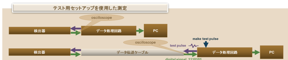
図 4.17 出力波形を観測するセットアップの概略図
