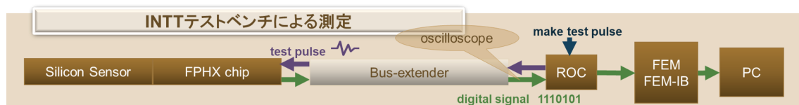
図 3.2 テストベンチの概略図
