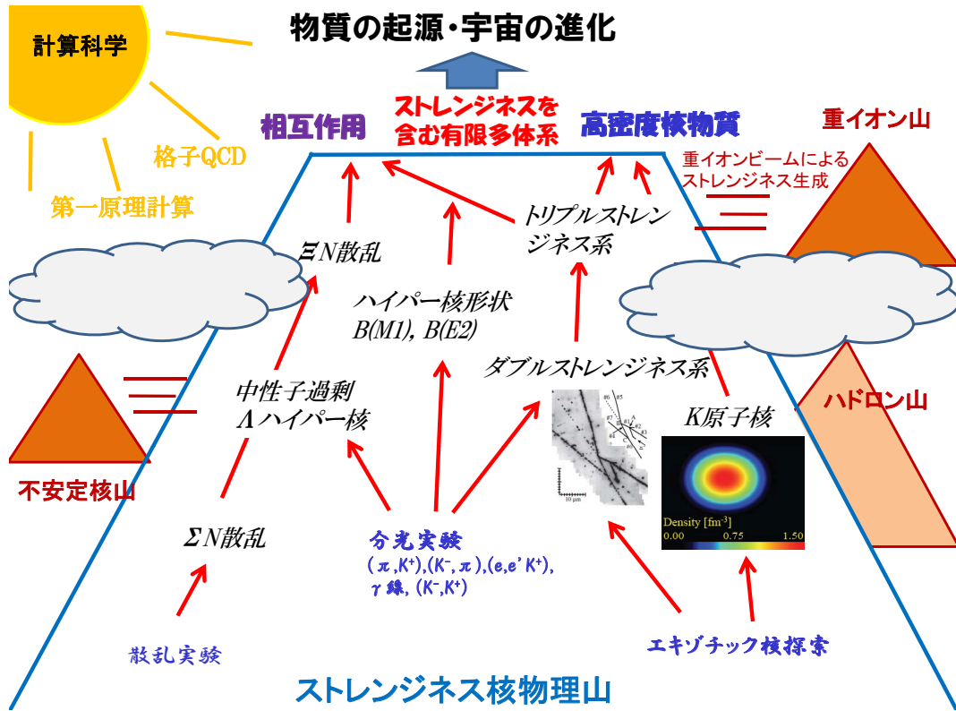
図 13: ストレンジネス核物理の今後の発展を示す図。
