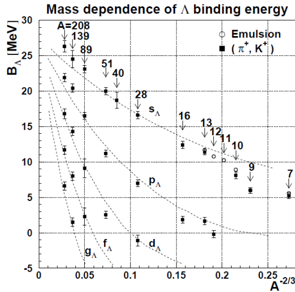
図 4: \Lambda 束縛エネルギーの質量数依存性。
