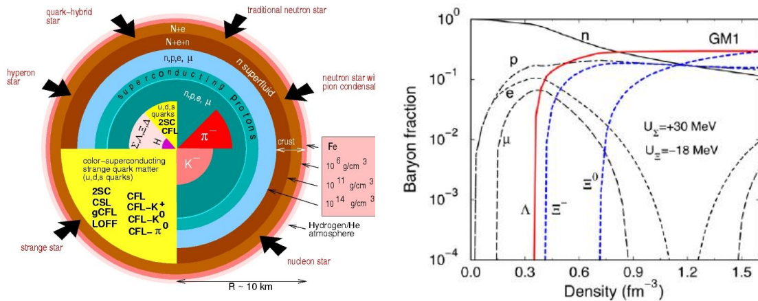
図 3: (左) F. Weber による中性子星内部構造。どのような模型 (状態方程式) をとるかによって、コアの物質形態は異なる。(右) GM1 セットをもちいた平均場計算による中性子星物質中でのバリオンの存在割合と密度の関係。ハイペロンのポテンシャルは -29 \text{ MeV}(\Lambda) , +30 \text{ MeV}(\Sigma) , -18 \text{ MeV}(\Xi) で、 YY 間相互作用は小さいと仮定している [2]。
