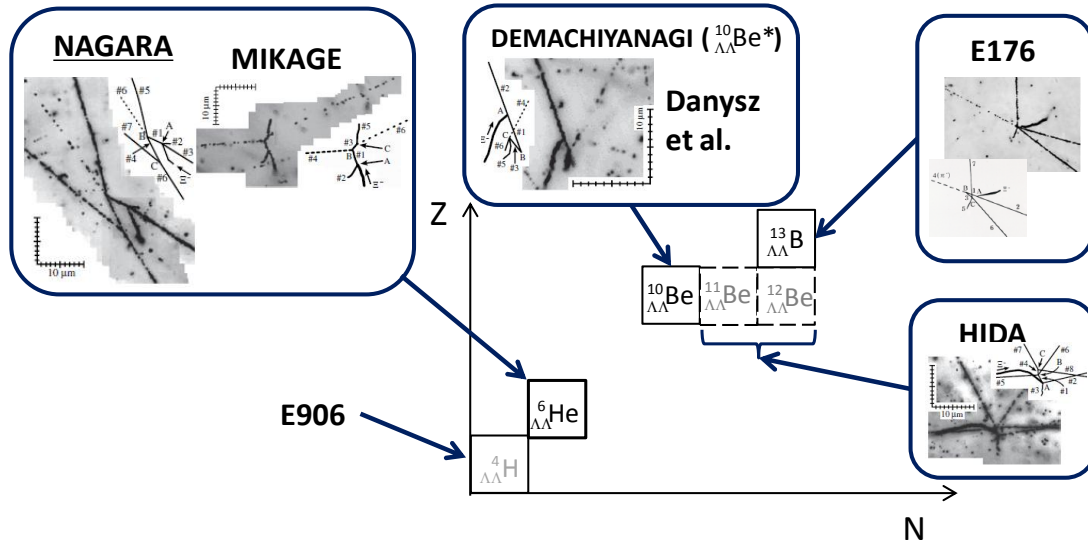
図 9: \Lambda\Lambda 核の核図表。実験で曖昧さなく同定されているのは、NAGARA と名付けられた事象 ( {}^6_{\Lambda\Lambda}\text{He} ) のみである。
