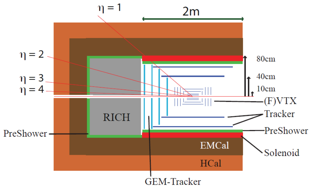
図 12: PHENIX 実験の検出器高度化の計画 (sPHENIX 計画)。
