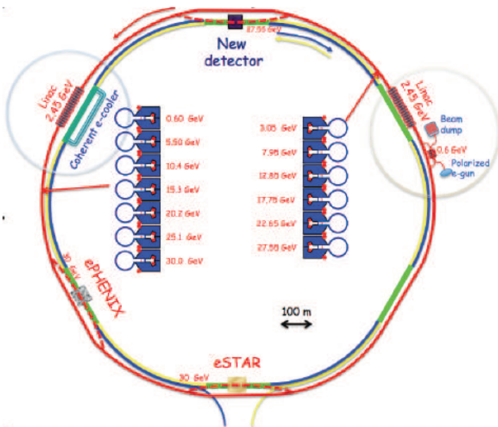
図 16: eRHIC の見取り図。
