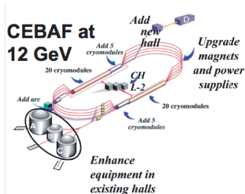
図 13: JLab 12GeV アップグレード計画のコンセプト。
