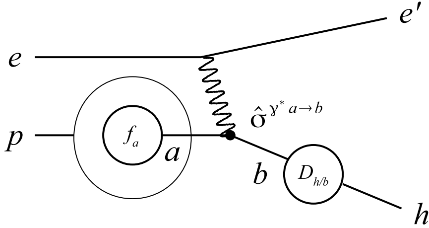
図 3: SIDIS 過程
