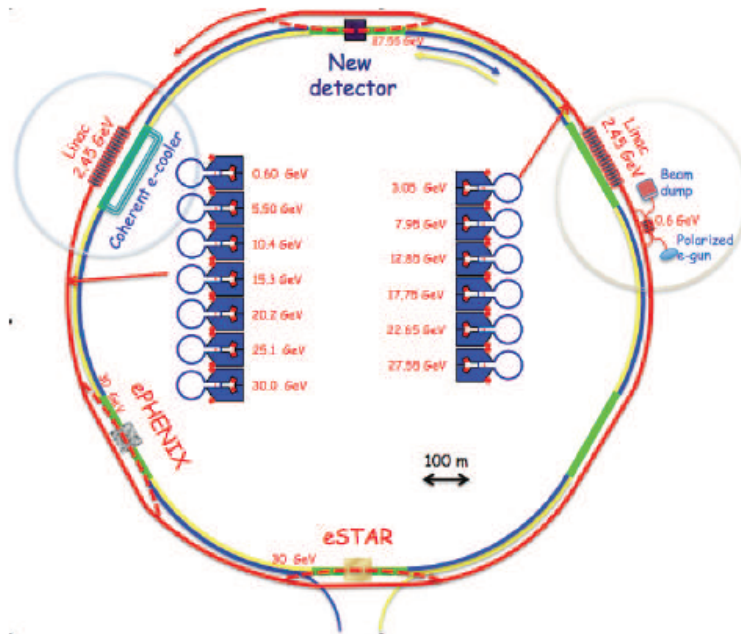
図 17: eRHIC の見取り図。
