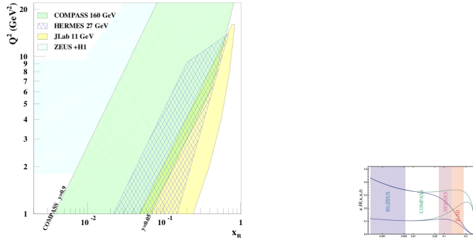
図 14: DVCS 実験での運動学的測定領域
