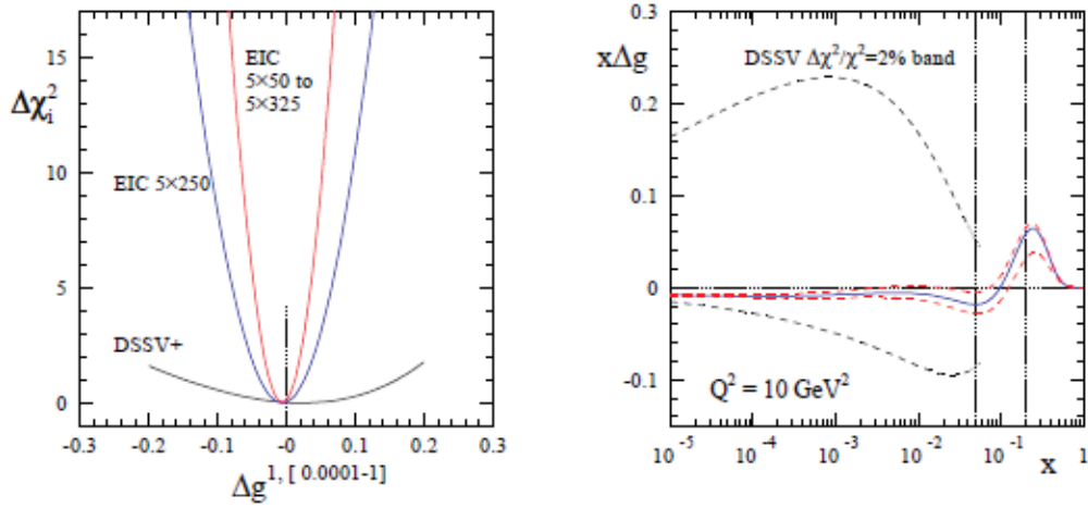
図 13: EIC で得られる \Delta G(x) の精度。
