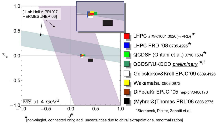
図 9: 核子内でのアップクォーク・ダウクォーク全角運動量 [42]。
