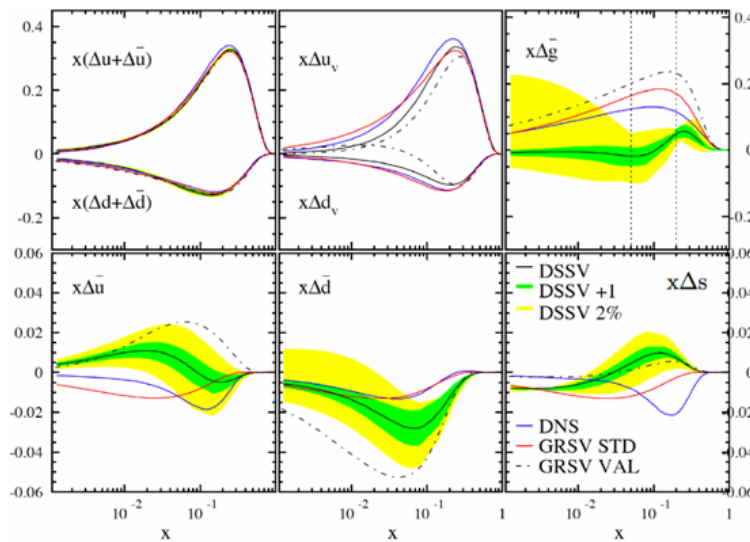
図 6: QCD グローバル解析の結果得られている偏極クォーク、反クォーク、グルーオン分布関数。
