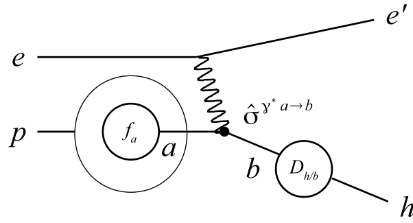
図 4: SIDIS 過程
