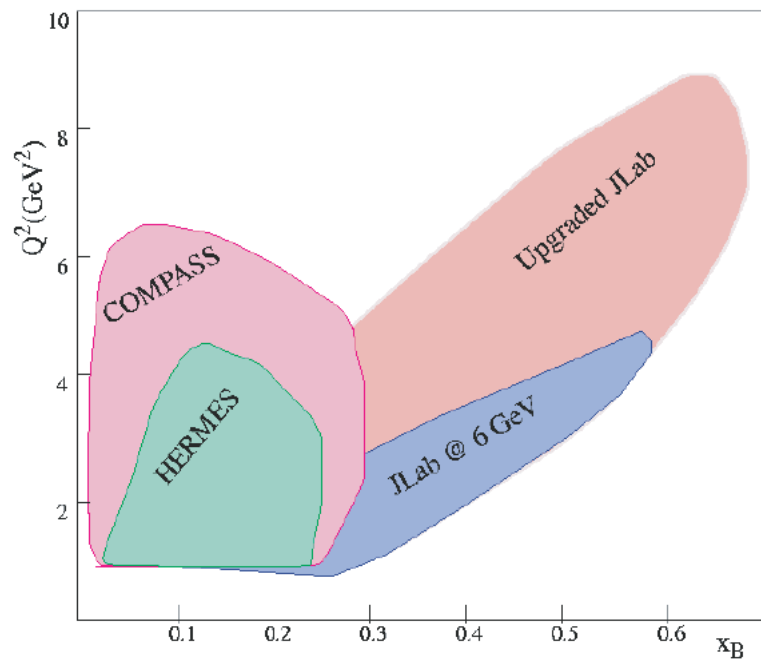
図 16: 異なる実験施設における深非包括運動学のカバー範囲。
