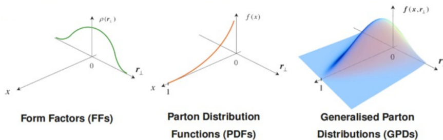
図 8: 一般化パートン分布とパートン分布・形状因子
