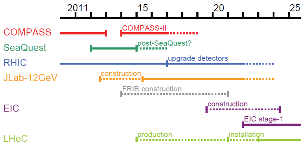
図 18: 今後の実験計画のタイムライン。
