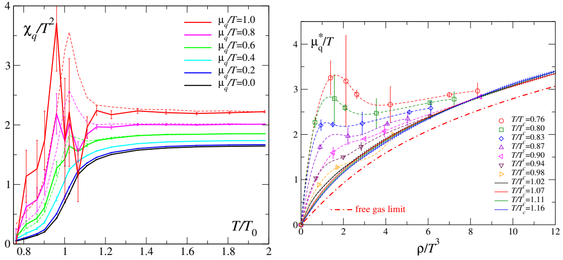
図5 (左図) 級数展開法で計算したクォーク数の揺らぎの温度 ( T ) 依存性 [27]。有限化学ポテンシャル ( \mu_q ) での臨界点でこの量は発散すると考えられている。実線は O(\mu_q^4) まで、破線は O(\mu_q^2) まで考慮。 T_0 は \mu_q = 0 での相転移温度。(右図) カノニカル分配関数から計算した化学ポテンシャル \mu_q^* とクォーク数密度 \rho の関係。温度が低いところでは一つの化学ポテンシャルに対して密度は複数の値を取りえることを示している。これは一次相転移点での二相共存に対応し、低温高密度領域に一次相転移があることを示唆している [28]。
