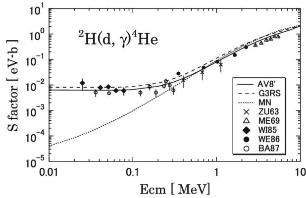
図6 現実的核力 (AV8' および G3RS) を用いて計算された {}^2\text{H}(d, \gamma){}^4\text{He} 反応の Astrophysical S factor を、実験値と比較した図、有効中心力のみを含む核力ポテンシャル (MN) を用いた場合と比べて、低エネルギー領域で S factor がほとんど減少せず、水平になっていることがわかる。文献 [39] から引用。
