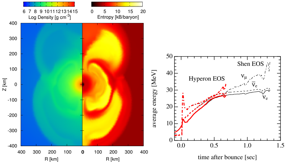
図9 (左図) 2次元(軸対称)の超新星数値シミュレーションにおける爆発の例を密度・エントロピーのカラーマップで示した。流体不安定性との組み合わせでニュートリノ加熱の効果があがり、コアバウンス後の長い時間を経てから爆発に至る計算例が示された。( [8] 参照。図は諏訪雄大氏提供。 ) (右図) 大質量星の重力崩壊からブラックホールに至るまでに放出されるニュートリノの平均エネルギーの時間変化を示した。核子物質 (Shen EOS) とハイペロン混入物質 (Hyperon EOS) の状態方程式を用いた数値シミュレーションでは、ニュートリノ放出の継続時間に大きな違いがあり、観測によりハイペロン出現をプローブできる可能性がある。( [63] 参照。 )
