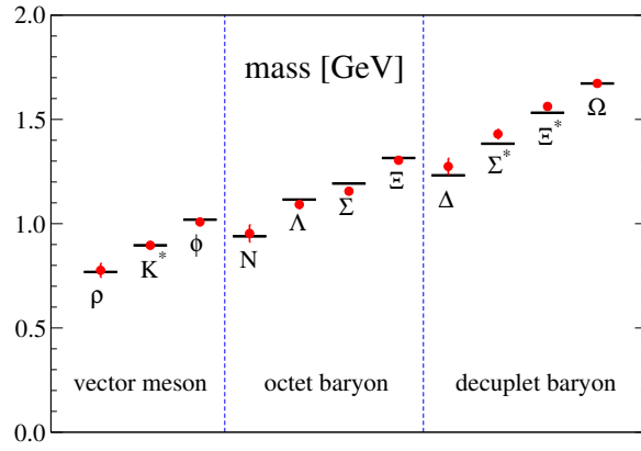
図 2 筑波大学 PACS-CS グループによる 2 + 1 フレーバ格子 QCD 計算による軽いハドロンの特クトルの結果。 m_\pi, m_K, m_\Omega の実験値をインプットとして使っている。文献 [2] より引用。
