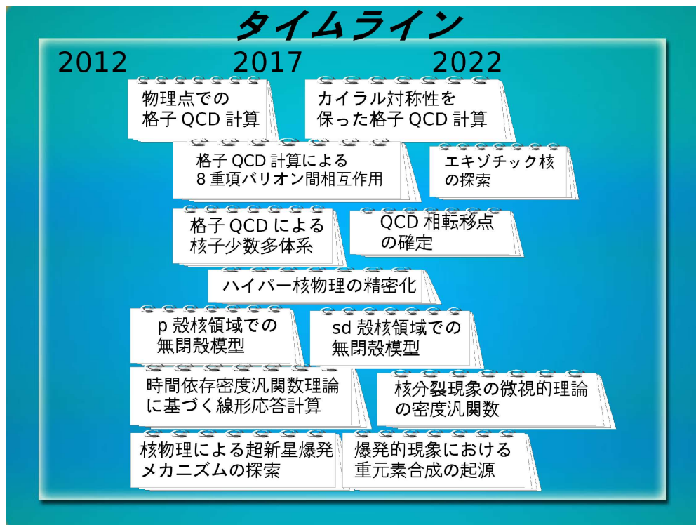
図 10 計算核物理で将来の課題として掲げた各課題のタイムラインを示す。
