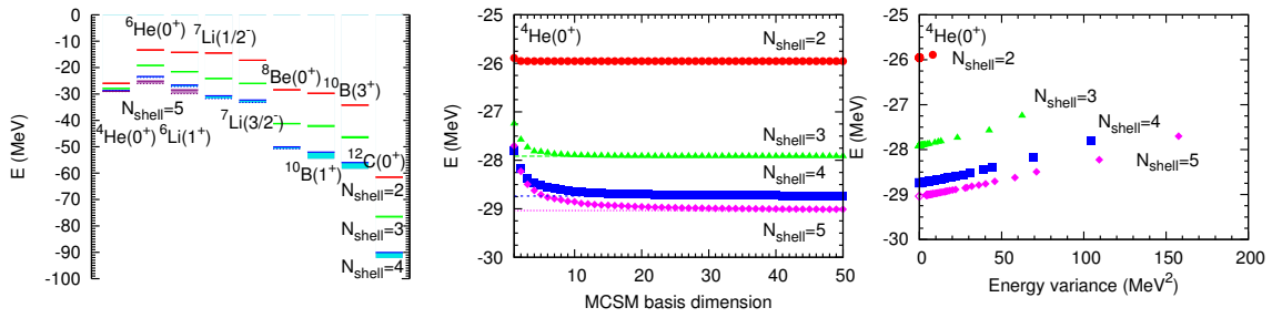
図 7 (左図) モンテカルロ殻模型を用いた第一原理計算による軽核のエネルギーのベンチマーク。実線がモンテカルロ殻模型計算、バンドがエネルギー分散による外挿からくる補正、点線が厳密解。 N_{\text{shell}} は模型空間の大きさを示す。文献 [5] 参照。(中央図) モンテカルロ殻模型計算によるエネルギーと基底数の関係。典型例としてヘリウム 4 原子核の基底状態 ( 0^+ ) を示す。点線は厳密解。(右図) 中央図の例に対応した基底数によるエネルギー分散の変化。エネルギー分散が 0 のところにある白抜きのシンボルは厳密解を示す。
