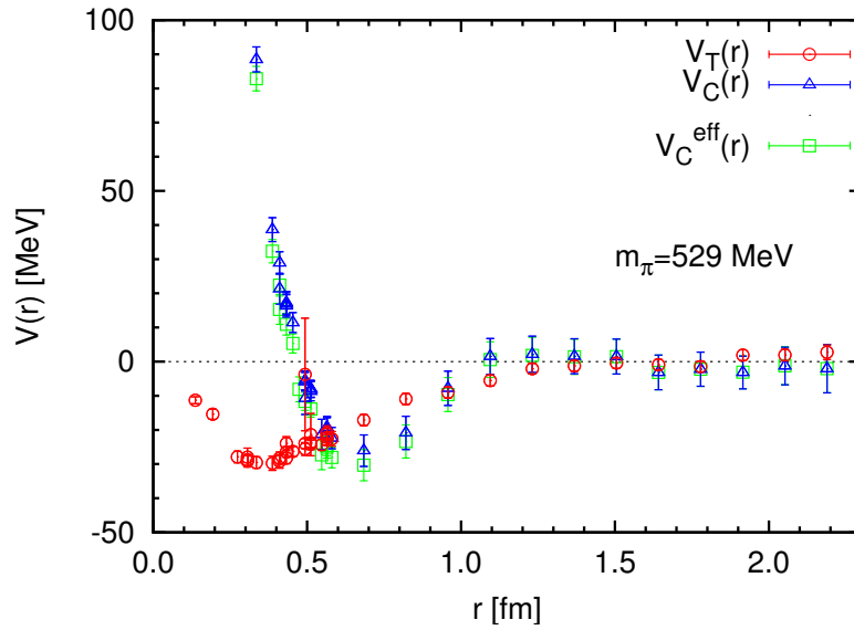
図3 \pi 中間子の質量が 529 MeV に相当するクォーク質量での、クエンチ近似の格子 QCD 計算で得られた、スピン三重項状態に対する核力ポテンシャル。三角が中心力、丸がテンソル力であり、四角はテンソル力を繰り込んだ場合の有効中心力ポテンシャル。文献 [25] より引用。
