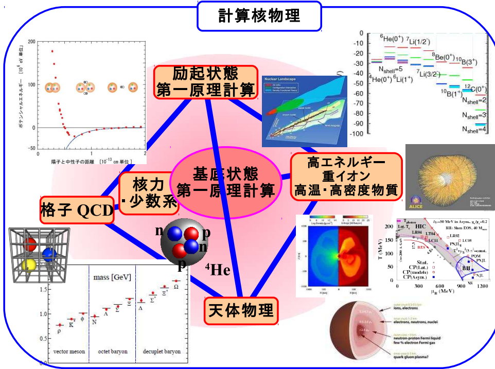
図 1 計算核物理が対象とする研究領域とそれぞれの相互の関係を模式的に示す。なかにはめ込んである図は、文献 [2, 3, 4, 5, 6, 7, 8, 9] から引用。
