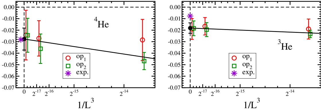
図4 クエンチ近似の格子 QCD 計算による軽い原子核、 {}^4\text{He} (左図)と {}^3\text{He} (右図)、の束縛エネルギーの計算。図では、原子核に対するエネルギーシフト \Delta E_n = M({}^n\text{He}) - nM(N) [GeV] の空間体積 L^3 依存性を 2 種類の生成演算子に対してプロットしている。黒丸と星印はそれぞれ空間体積無限大極限への外挿値と実験値を表す。文献 [26] 参照。
