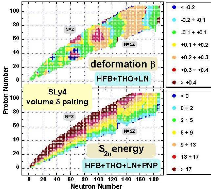
図8 汎用コードHFBTHOを用いた偶々核の四重極変形度 \beta (上のパネル)と二中性子分離エネルギー S_{2n} (数値の単位はMeV)(下のパネル)(文献[62]より引用)
