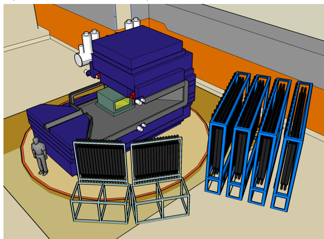
図 2.1.18: RIBF の SAMURAI スペクトロメータ。 中心に緑色で示したのが SAMURAI-TPC。
