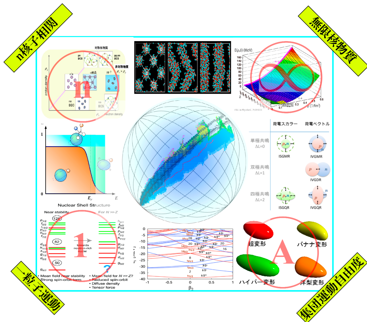
図 2.1.1: 不安定核分野の細分野分け。
