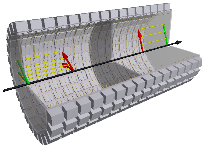
図 2.1.11: アクティブ標的。
