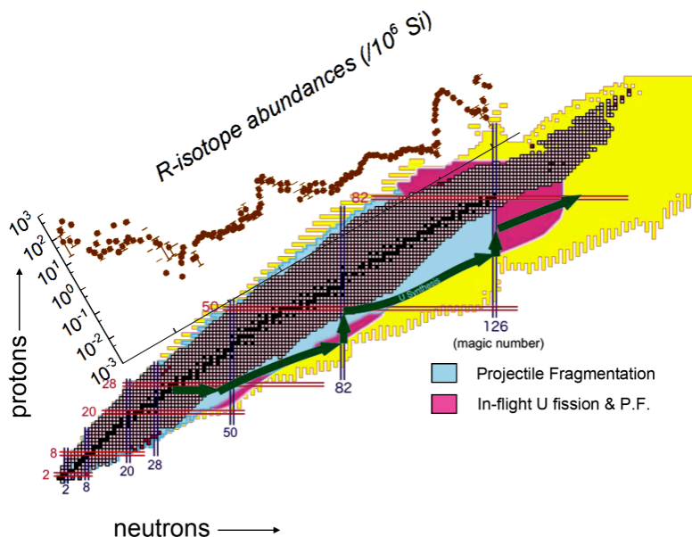
図 2.1.21: グリーン; 予想される r 過程経路。ピンク・ライトブルー; RIBF で 1 個/日以上生成率が期待される核種。
