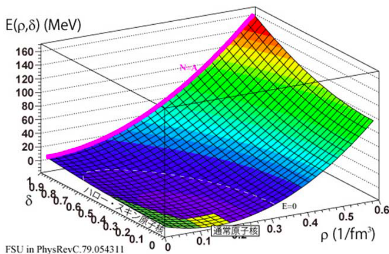
図 2.1.16: 状態方程式の例 [Pie09]。FSU と呼ばれるハイペロン構造を考慮していないもの。 N=A 、 \rho \gg \rho_0 の領域については外挿で、不確定性が大きい。
