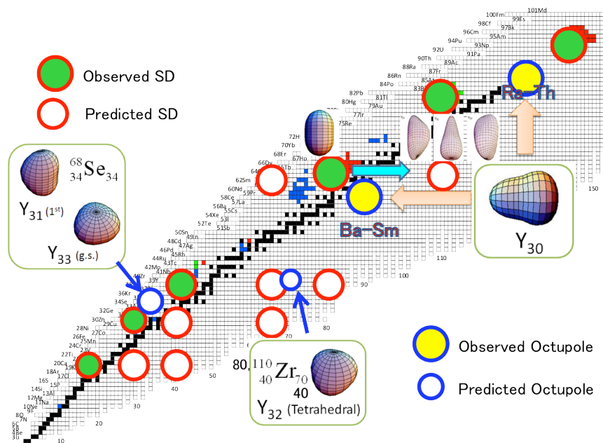
図 2.1.13: 核図表上に現れる様々な変形。
