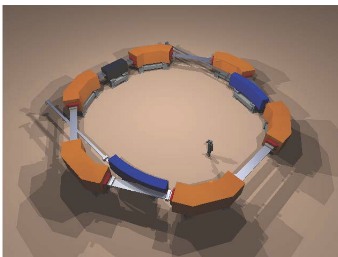
図 2.1.7: エネルギー補償型蓄積リングによる超希少核研究への挑戦。
