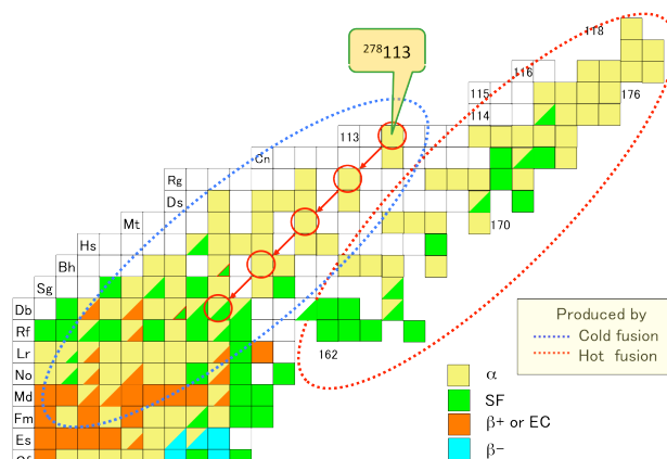
図 2.1.20: 超重核領域の核図表。
