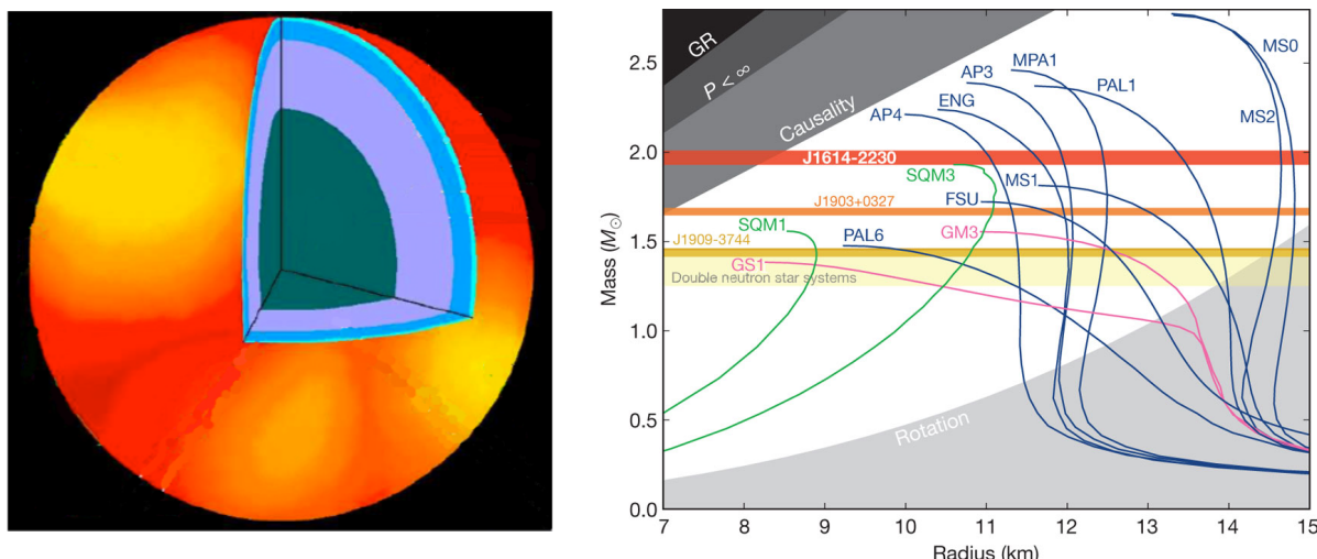
図 2.1.17: (左)中性子星の内部構造。外側から内側に向かって密度が上がり多彩な構造が存在すると考えられている。(右) 様々な EOS が予想する中性子星の質量と半径。青い線が中性子だけの場合、紫の線がハイペロン構造を考慮した場合、緑色の線が内部構造がクォークの場合を示す。[Dem10]
