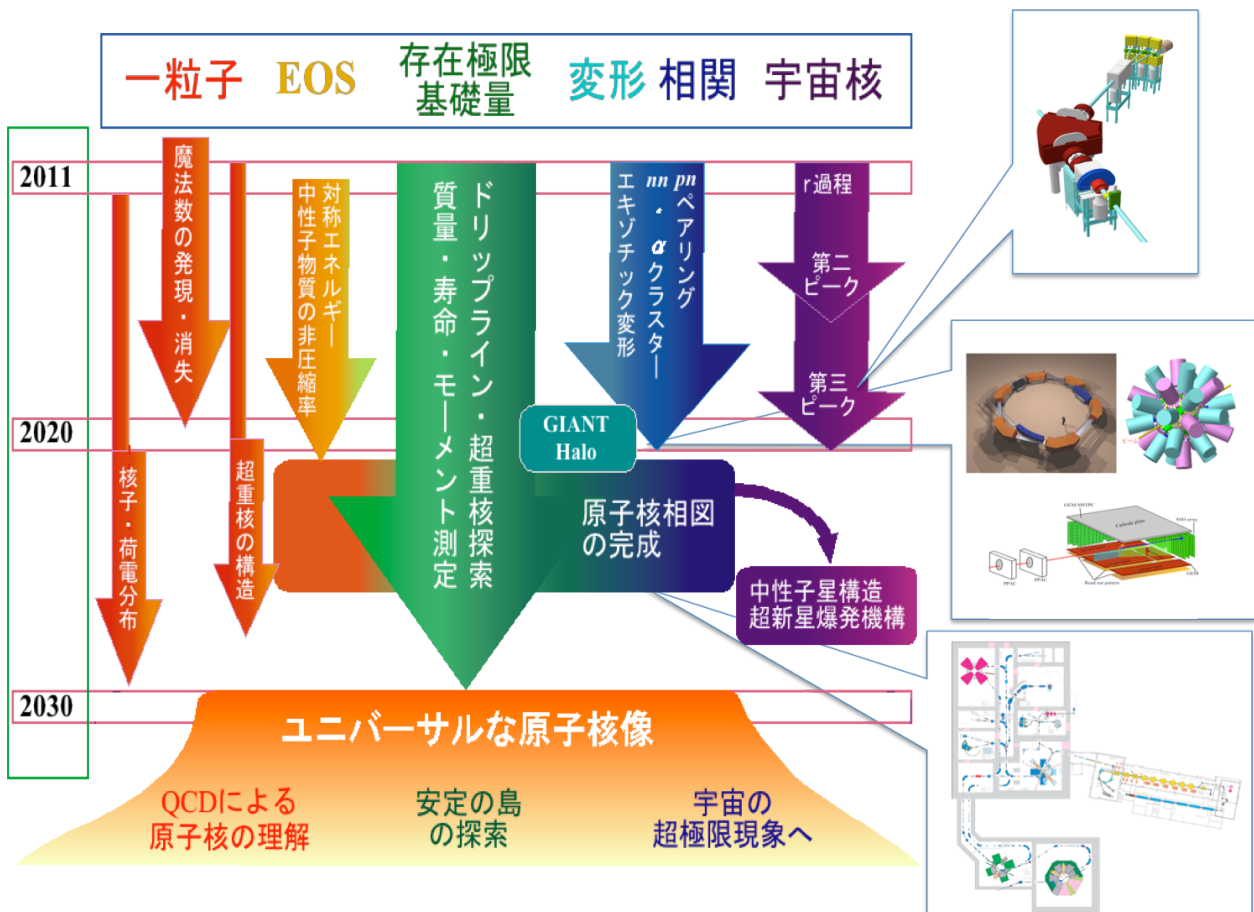
図 2.1.22: 不安定核研究タイムライン。
