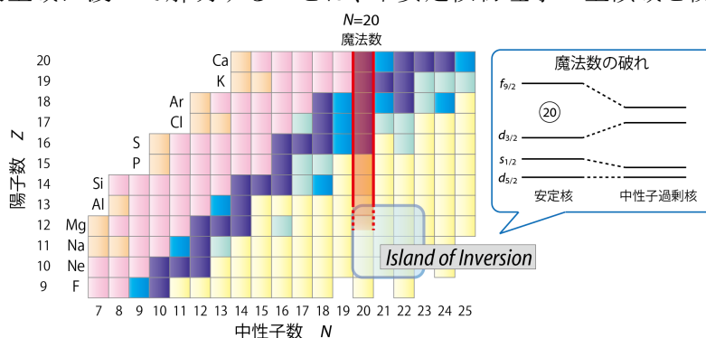
図 2.1.5: Island of Inversion 付近の核図表。
