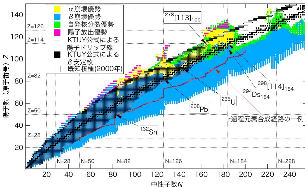
図 2.1.19: KTUY 質量公式による崩壊様式の予想図。
