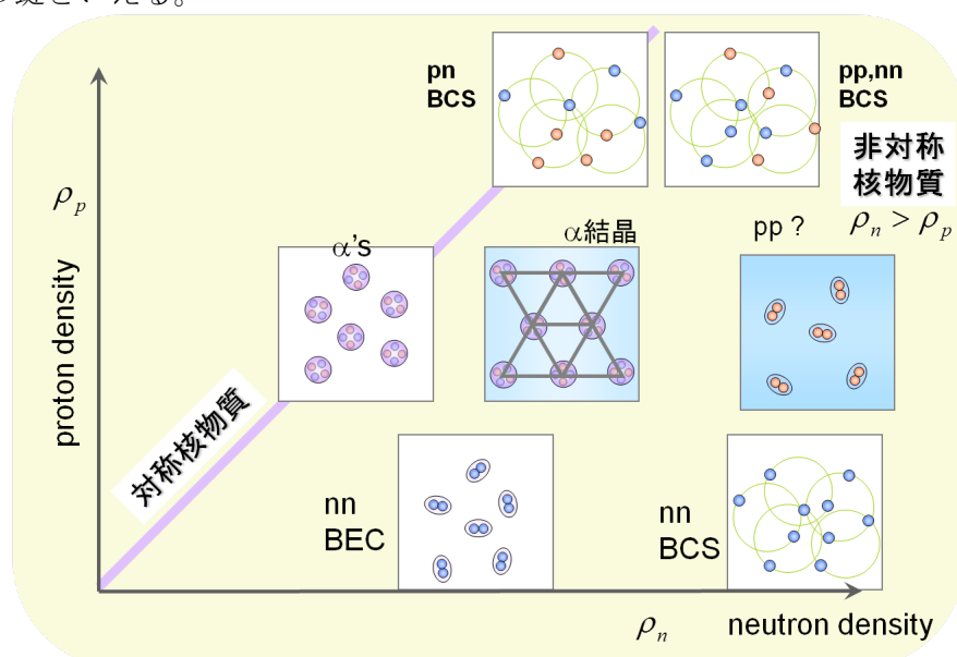
図 2.1.8: 中性子数と陽子数の変化によって出現する多様な原子核相。
