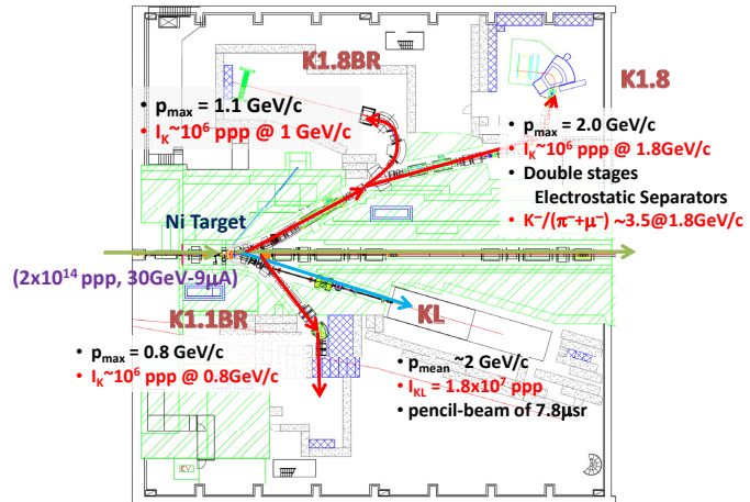
図 13: 2011 年現在の J-PARC ハドロン実験ホール。
