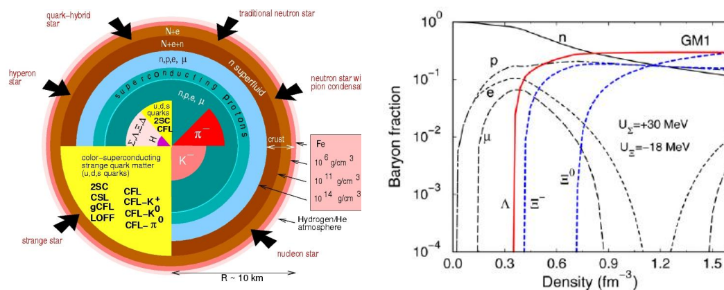
図 3: (左) F. Weber による中性子星内部構造 [2]。どのような模型 (状態方程式) をとるかによって、コアの物質形態は異なる。(右) GM1 セットをもちいた平均場計算による中性子星物質中でのバリオン及びレプトンの存在割合と密度の関係。ハイペロンのポテンシャルは -29 MeV ( \Lambda ), +30 MeV ( \Sigma ), -18 MeV ( \Xi ) で、 YY 間相互作用は小さいと仮定している [3]。
