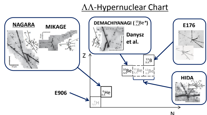
図 9: \Lambda\Lambda 核の核図表。実験で曖昧さなく同定されているのは、NAGARA と名付けられた事象 ( {}^6_{\Lambda\Lambda}\text{He} ) のみである。
