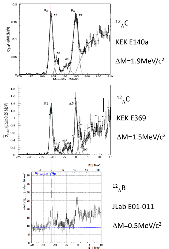
図 5: 分解能向上により、測定スペクトルがどのように変わるかを示す図。どれも ^{12}\text{C} を標的とした \Lambda ハイパー核の生成スペクトルである。(上) (\pi^+, K^+) 反応による ^{12}_{\Lambda}\text{C} スペクトル。分解能は 1.9 \text{ MeV}/c^2 (FWHM)[12]。(中) (\pi^+, K^+) 反応による ^{12}_{\Lambda}\text{C} スペクトル。分解能は 1.5 \text{ MeV}/c^2 (FWHM)[14]。(下) (e, e' K^+) 反応による ^{12}_{\Lambda}\text{B} スペクトル。分解能は 0.5 \text{ MeV}/c^2 (FWHM)[19]。
