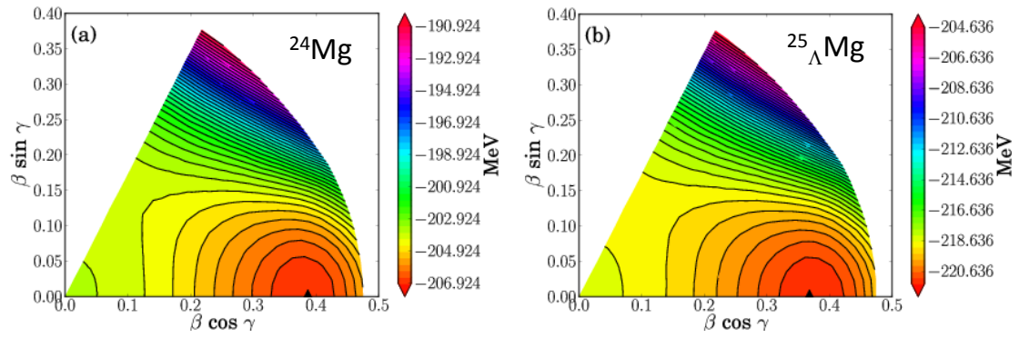
図 8: Skyrme Hartree-Fock + BCS 計算による ^{24}\text{Mg} 及び ^{25}_{\Lambda}\text{Mg} の Potential Energy Surface (PES)[78]。この図において、動径は、 \beta 方向の変形度、偏角は \gamma 方向の変形度を表す。ポテンシャル極小値を三角印で示す。 \Lambda 粒子が加わることで、極小値が \beta の小さい値にシフトし、PES が \gamma 方向にソフト化している。
