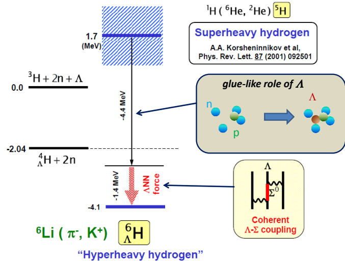
図 6: {}^6_{\Lambda}\text{H} 基底状態のエネルギー。非束縛のコア核 {}^5\text{H} に \Lambda を加えると \Lambda の glue-like role とコヒーレント \Lambda N - \Sigma N 結合で \sim 4 MeV の束縛となる [76]
