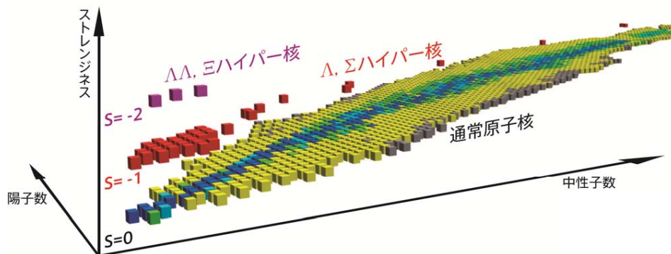
図 1: ストレンジネス自由度を加えた三次元核図表。
