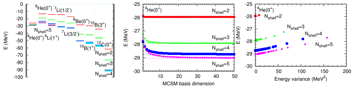
図 2.8.8 (左図) モンテカルロ殻模型を用いた第一原理計算による軽核のエネルギーのベンチマーク。実線がモンテカルロ殻模型計算、バンドがエネルギー分散による外挿からくる補正、点線が厳密解。 N_{\text{shell}} は模型空間の大きさを示す。文献 [6] 参照。(中央図) モンテカルロ殻模型計算によるエネルギーと基底数の関係。典型例としてヘリウム 4 原子核の基底状態 ( 0^+ ) を示す。点線は厳密解。(右図) 中央図の例に対応した基底数によるエネルギー分散の変化。エネルギー分散が 0 のところにある白抜きのシンボルは厳密解を示す。
