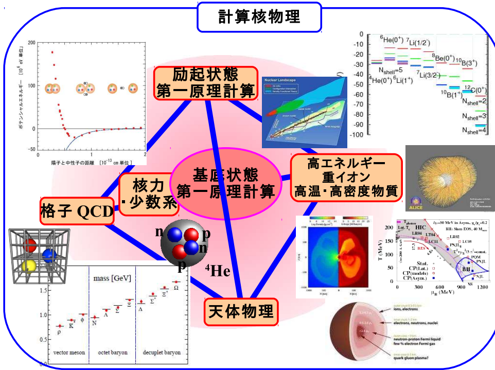
図 2.8.1 計算核物理が対象とする研究領域とそれぞれの相互の関係を模式的に示す。なかにはめ込んである図は、文献 [3, 4, 5, 6, 7, 8, 9, 10] から引用。
