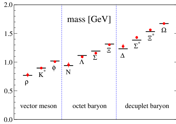
図 2.8.2 筑波大学 PACS-CS グループによる 2 + 1 フレーバ格子 QCD 計算による軽いハドロンのスペクトルの結果。 m_\pi, m_K, m_\Omega の実験値をインプットとして使っている。文献 [3] より引用。
