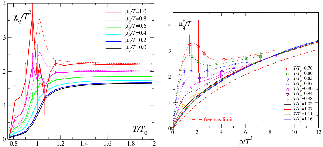
図 2.8.5 (左図) 級数展開法で計算したクォーク数の揺らぎの温度 ( T ) 依存性 [28]。有限化学ポテンシャル ( \mu_q ) での臨界点でこの量は発散すると考えられている。実線は O(\mu_q^4) まで、破線は O(\mu_q^2) まで考慮。 T_0 は \mu_q = 0 での相転移温度。(右図) カノニカル分配関数から計算した化学ポテンシャル \mu_q^* とクォーク数密度 \rho の関係。温度が低いところでは一つの化学ポテンシャルに対して密度は複数の値を取りえることを示している。これは一次相転移点での二相共存に対応し、低温高密度領域に一次相転移があることを示唆している [29]。
