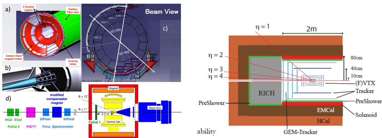
図 2.5.26: 次世代 PHENIX 検出器 (sPHENIX) の計画 [32]
