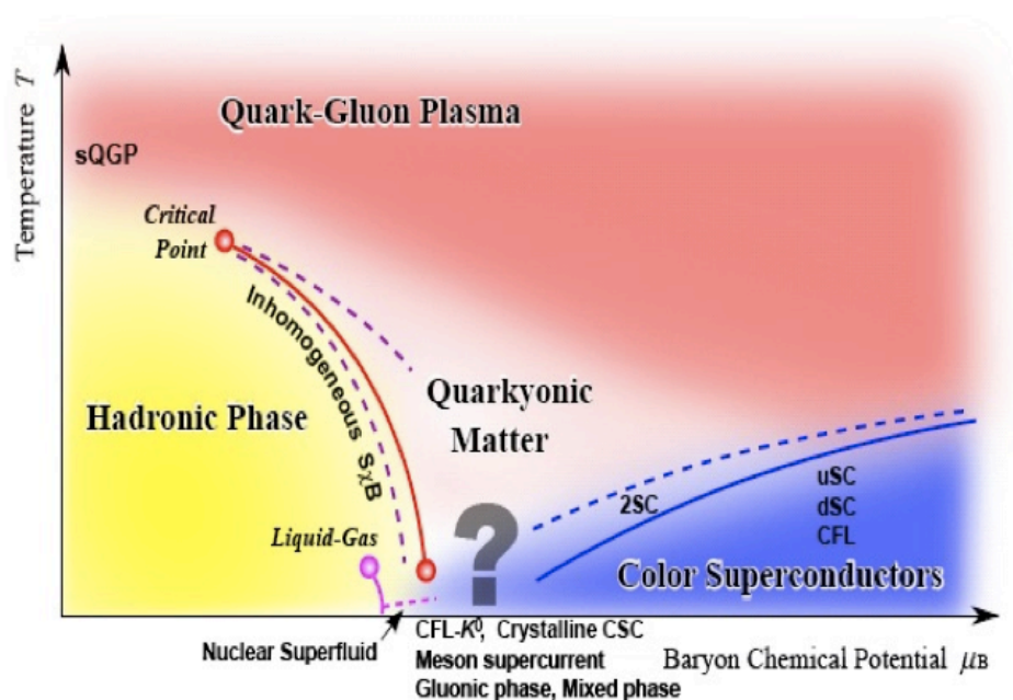
図 2.5.1: QCD 相図の温度やバリオン化学ポテンシャル依存性 [1]
