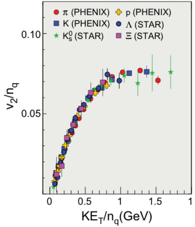
図 2.5.9: v_2 のハドロン構成数でのスケーリング [9]
